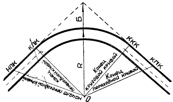
Рис. 60. Знаки начала и конца кривых
