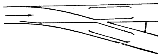
Рис. 26. Противощерстная стрелка
