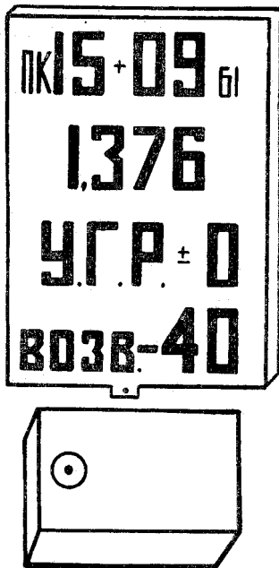
Рис. 59. Реперный знак
