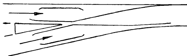
Рис. 25. Пошерстный стрелочный перевод
