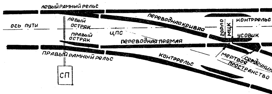
Рис. 24. Стрелочный перевод
