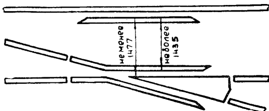
Рис. 47. Контрольные размеры 1477 и 1435
