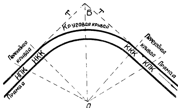
Рис. 53. Круговая кривая
