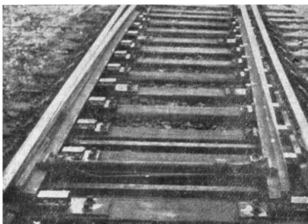
Рис. 29. Стрелочные подушки
