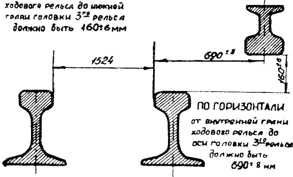
Рис. 66. Габаритные размеры 3-го рельса
