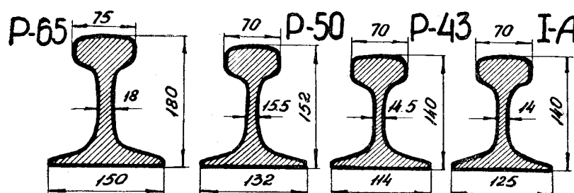
Рис. 8. Типы рельсов
