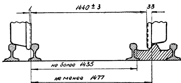
Рис. 49. Положение колесной пары на крестовине
