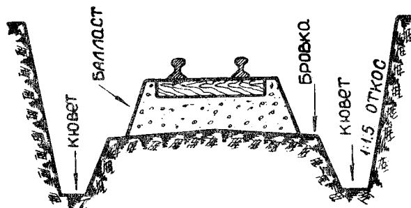
Рис. 2. Выемка
