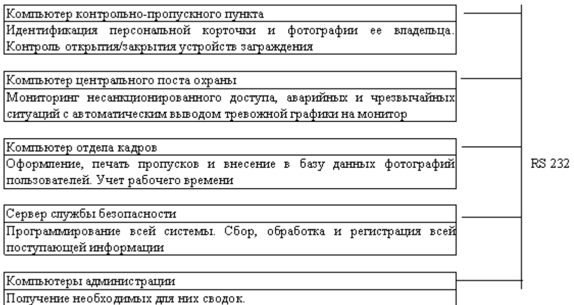
Рисунок 7 - Примерное размещение компьютеров СКУД, объединенных в сеть, на объекте
